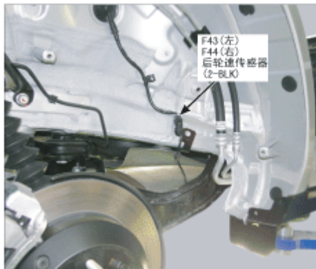
130. 后轮壳
