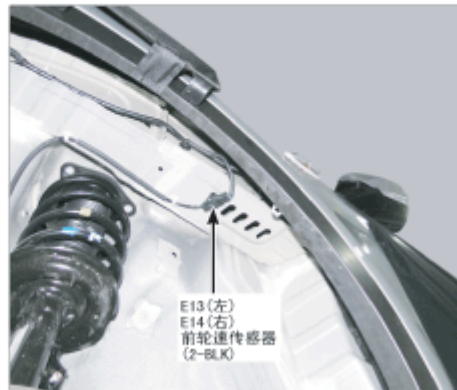
129. 前轮壳
