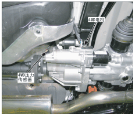
127. 后悬架前部
